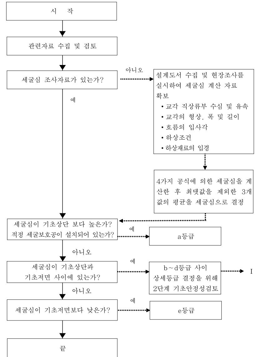
[그림 1.3] 1단계 세굴심 평가 결과 산정 방법
