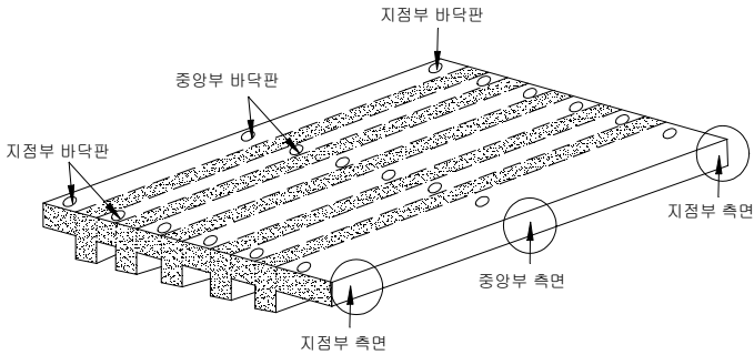
< 거더가 있는 경우의 바닥판점검부위 >
