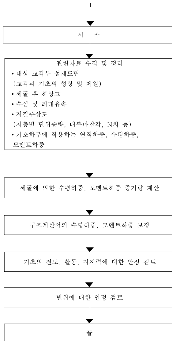
[그림 1.4] 2단계 기초안정성 평가 결과 산정 방법
