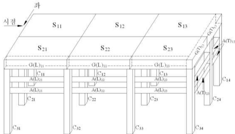
[그림 1.2] 라멘교의 부재 구성도
