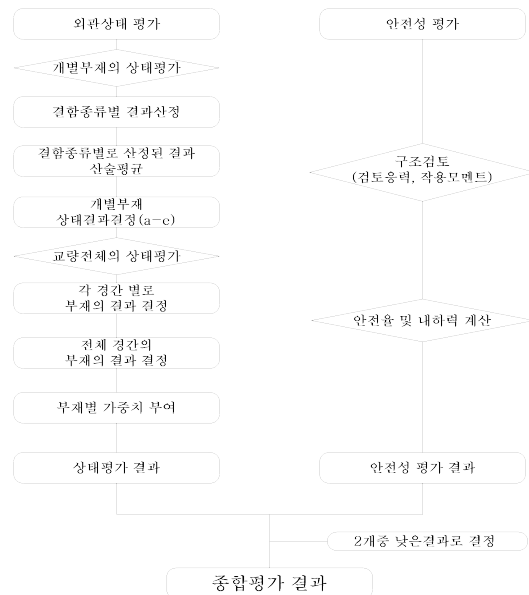
[그림 1.5] 종합평가결과의 산정 흐름도
