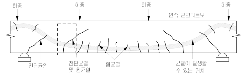
< 콘크리트 거더에 발생하는 균열의 유형과 위치 >
