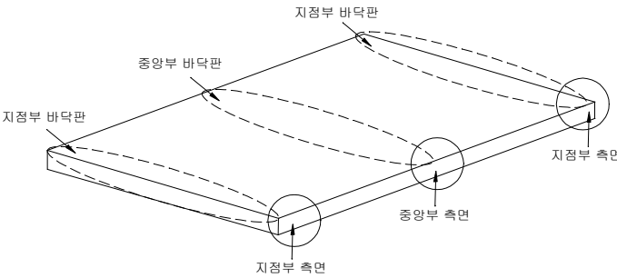
< 거더가 없는 경우의 바닥판 점검부위 >
