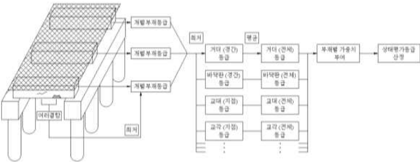
[그림 1.1] 전체 교량의 상태평가결과 산정 방법 예
